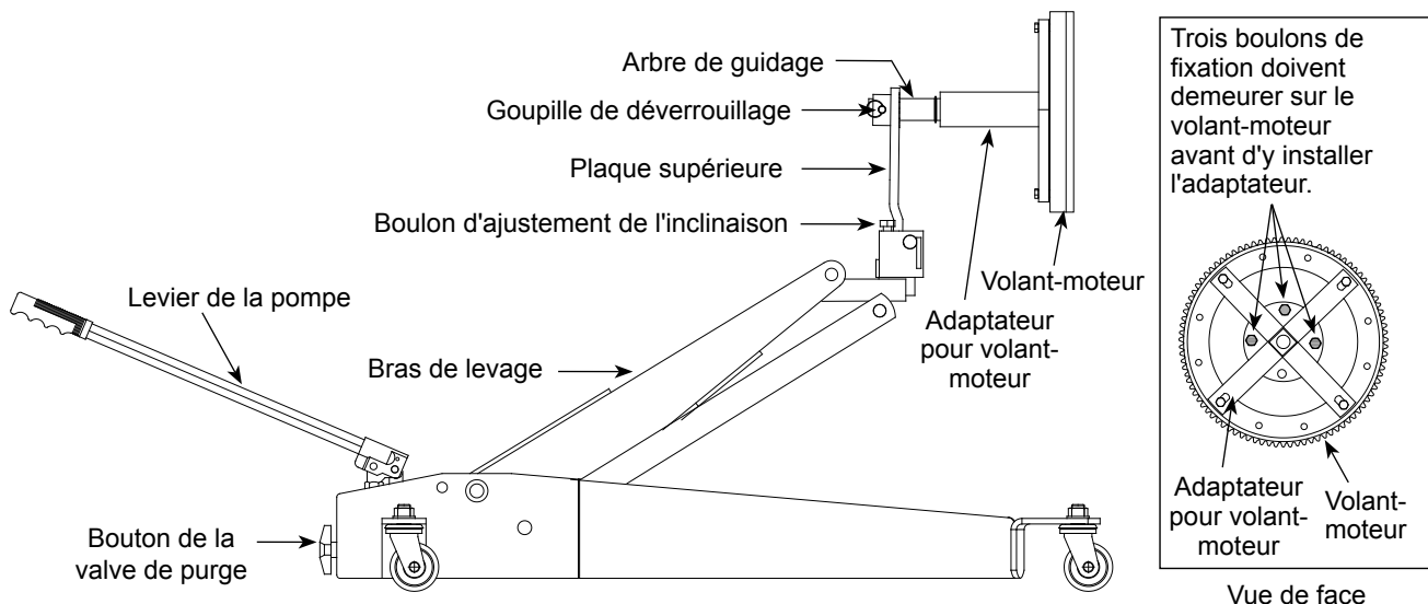
Figure 4 : Illustration d'utilisation de l'adaptateur pour volant-moteur
