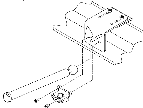
Figure 4 : Fixation du support à rotule et du bras de support à la plaque avant.
