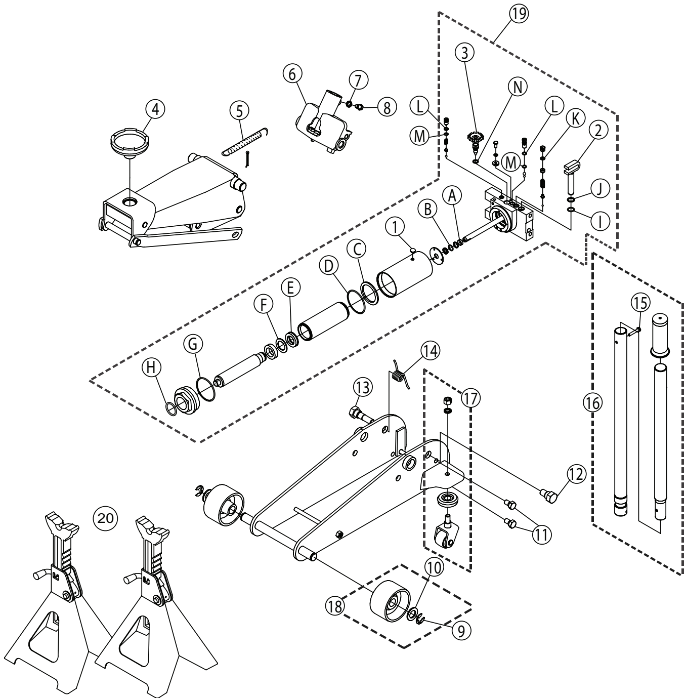
Figura 3: ilustración de piezas de repuesto para el gato de servicio combinado modelo BH6033
