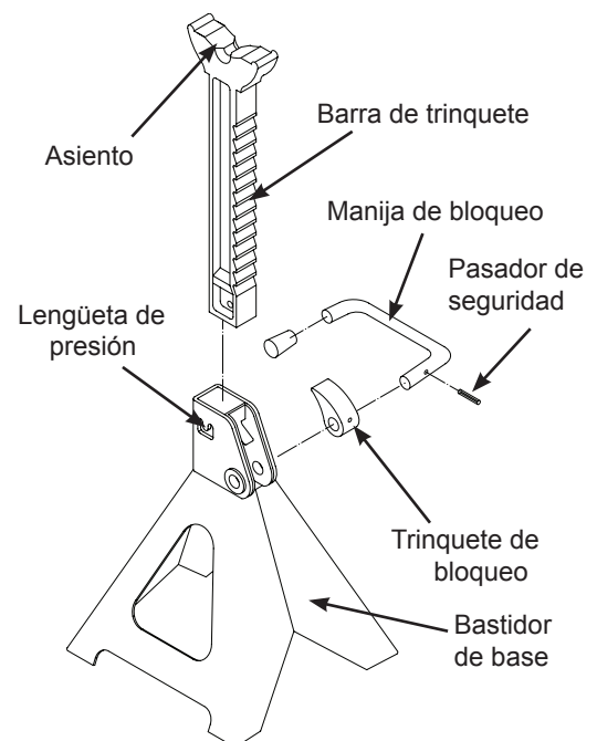
Figura 2: Componentes de un soporte para gato
