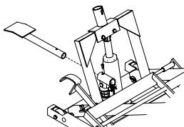
Figura 7: ensamblaje del pedal accionado por el pie.
